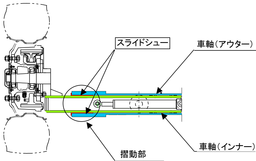
伸縮車軸断面図
